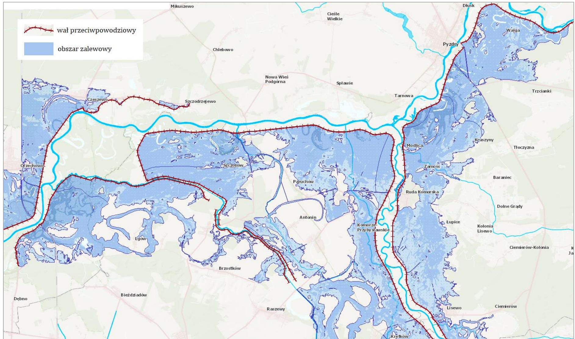
Rysunek 20. Przebieg wałów przeciwpowodziowych na terenie Powiatu Wrzesińskiego oraz obszary zalewowe dla scenariusza przerwania wałów przeciwpowodziowych
