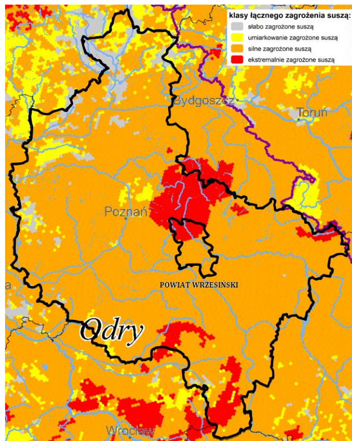
Rysunek 16. Łączne (wynikowe) zagrożenie Powiatu Wrzesińskiego suszą Źródło: „Projekt planu przeciwdziałania skutkom suszy” (Warszawa, październik 2020 r.)
