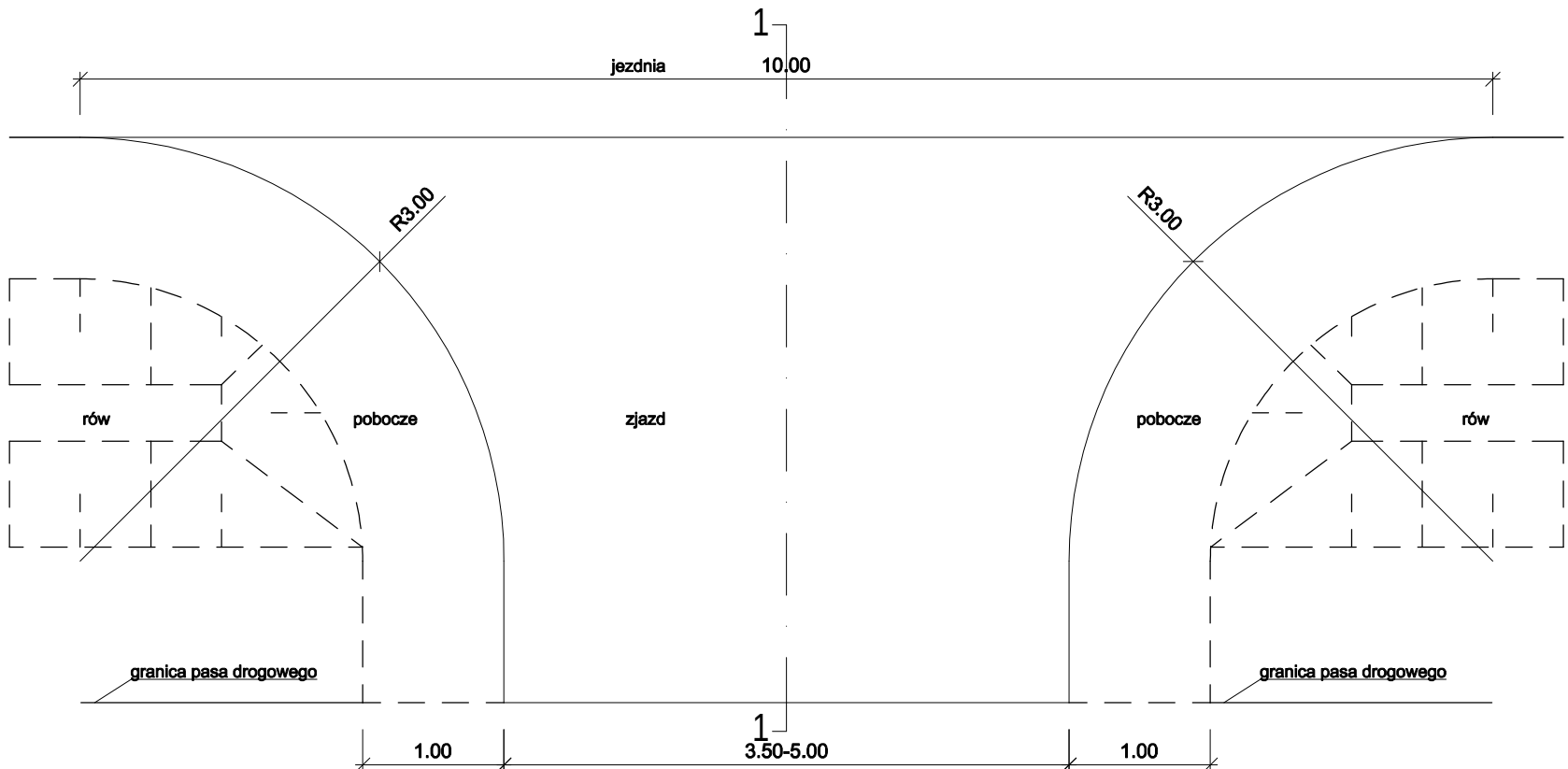
Przekrój 1-1 zgodnie z rys. 2.1-2.5
